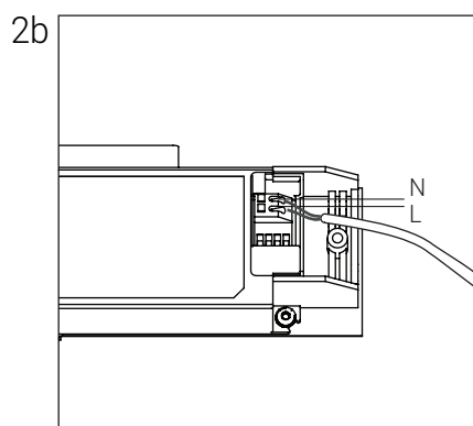
Схема подключения
